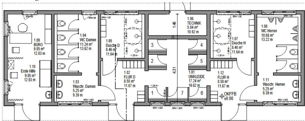
Abbildung 1: Grundriss Sanitärtrakt
