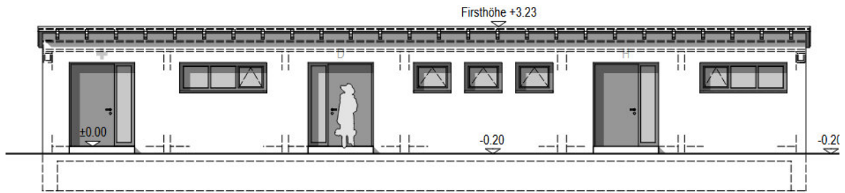
Abbildung 2: Planansicht Neubau Sanitärtrakt
